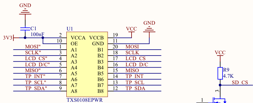
TXS0108EPWR
