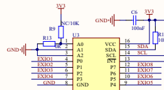
I/O Extensions
