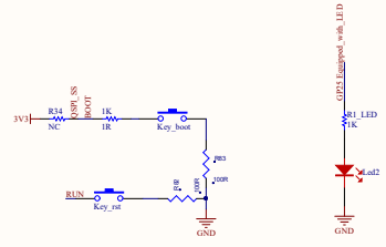
pico_RST pico_BOOT 按键
