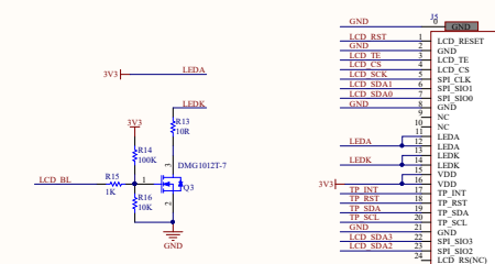
板对板连接器 0.4mm 24P 高0.8mm 母座 YXT
