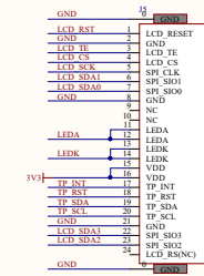
板对板连接器 0.4mm 24P 高0.8mm 母座 YXT
