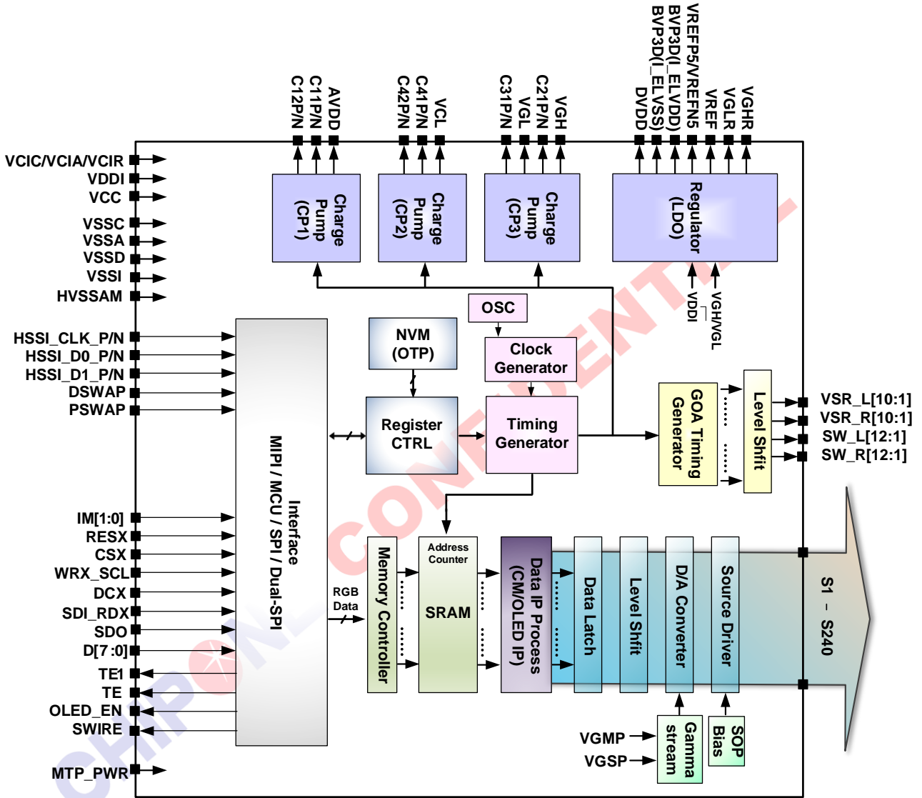
CO5300 Block diagram
